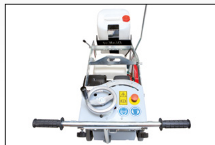
pohled obsluhy
