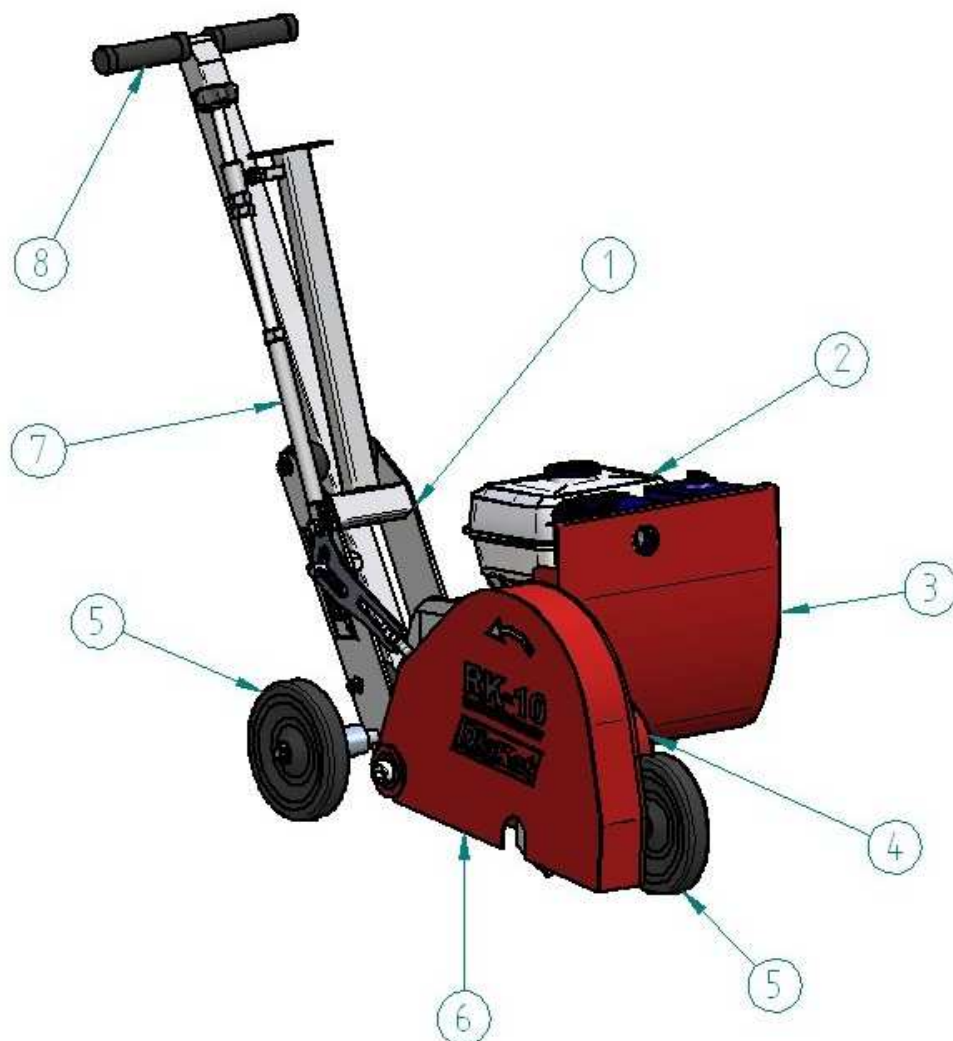
Obr. 1 Popis funkčních částí stroje
